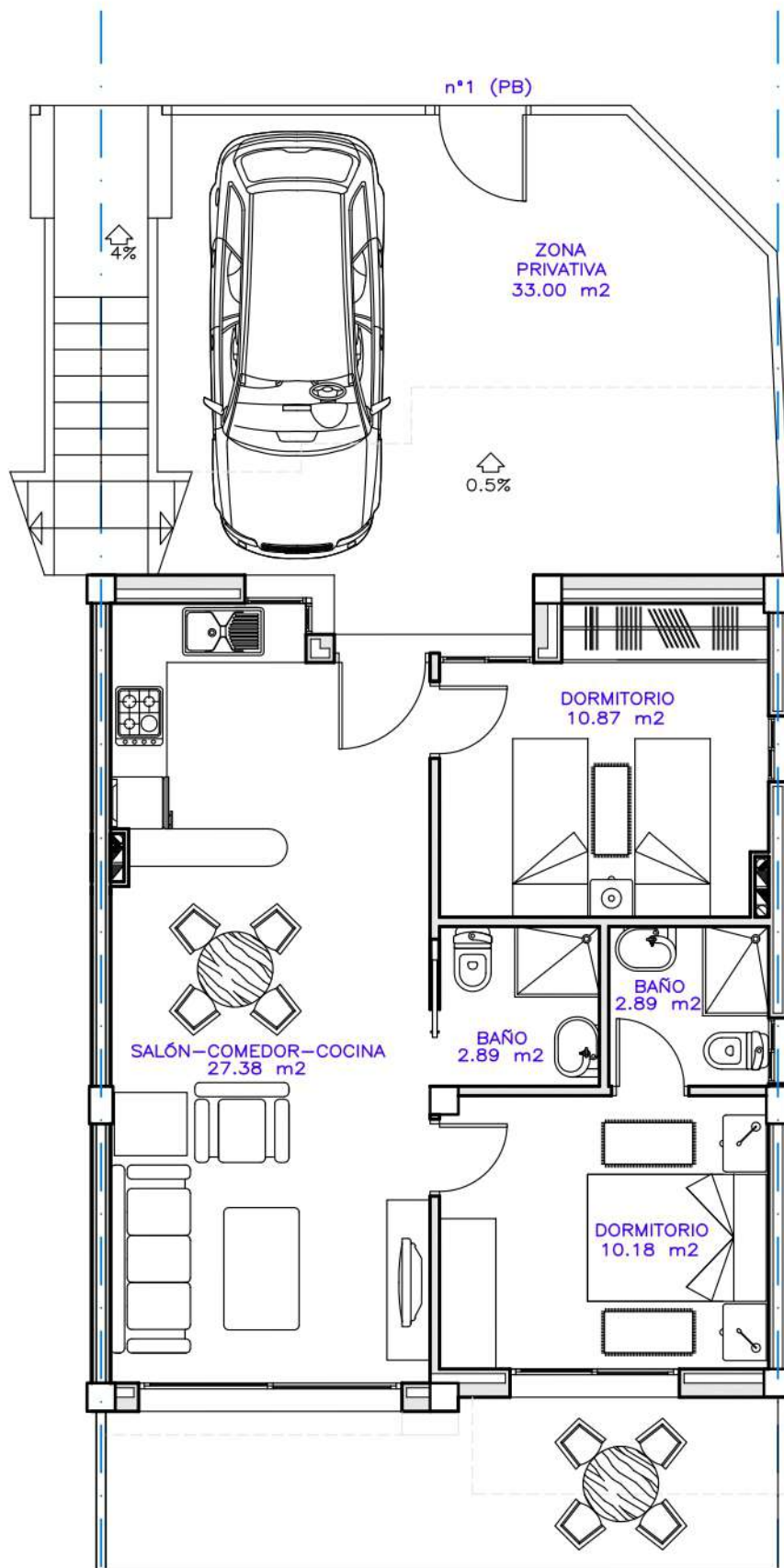
VIVIENDA PLANTA BAJA N° 1 ESQUINA
