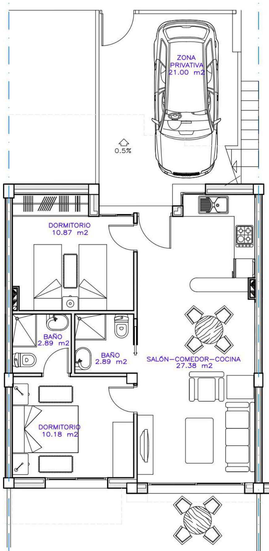
VIVIENDA PLANTA BAJA
